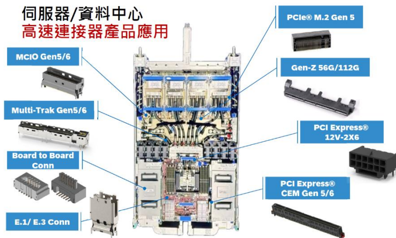
圖 3：宏致伺服器高速連接器產品應用圖
